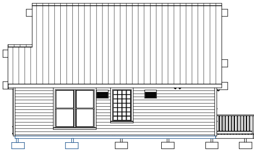
RIGHT ELEVATION
